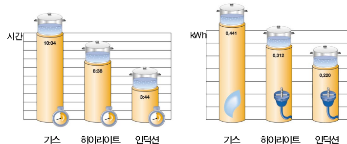
쿡탑 종류별 비교 - 2리터의 물을 끓일 경우 소요시간 및 에너지 소비량
